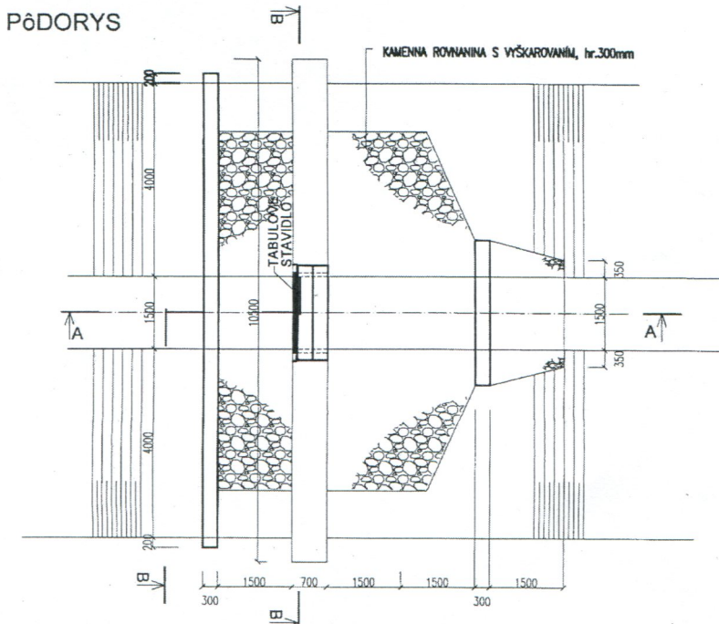
Obr. X.7. Tabuľové stavidlo (návrh)
