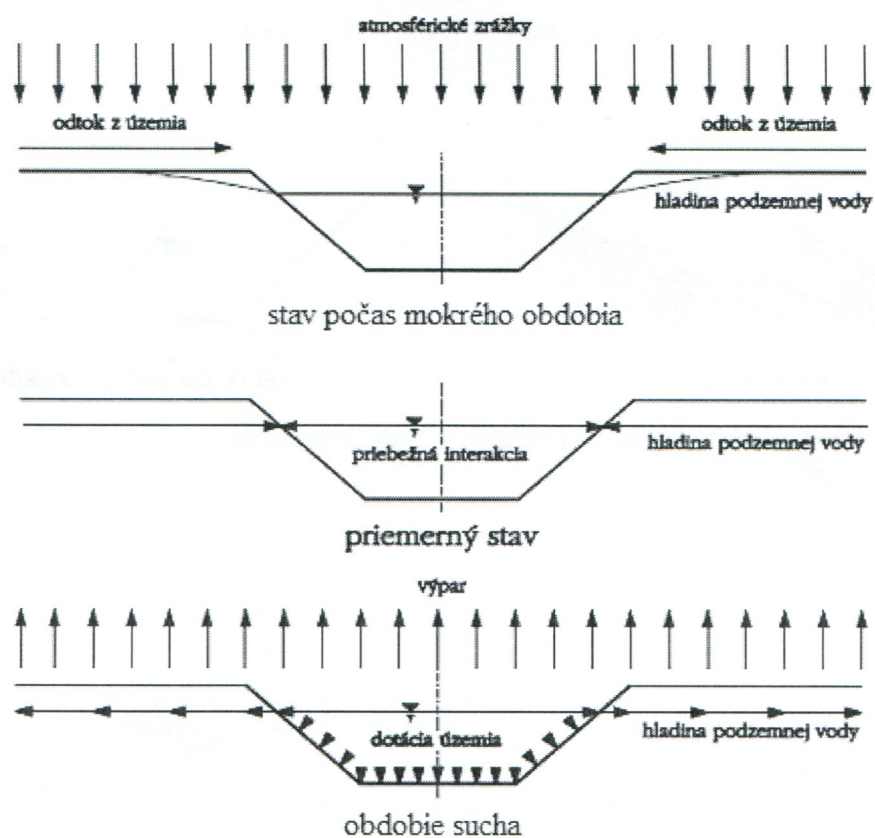
Obr. X.6. Schéma funkcie kanála počas vodného obdobia, priemerného stavu a obdobia sucha (priechy profil)
